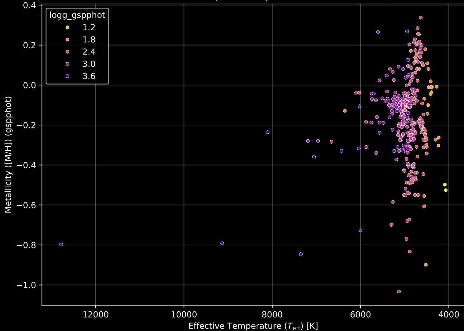
APOGEE DR17 Field: [hip] Stellar Population Parameters (n= 410)
